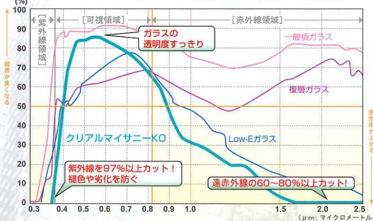
◆ グラフではっきり！可視光線透過率と熱線遮熱効果
